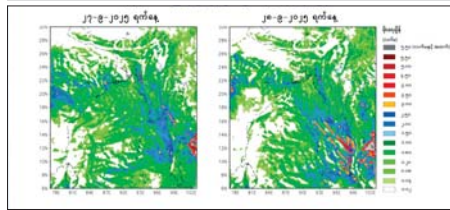
ယနေ့ညနေမှ ၃၀-၉-၂၀၂၅ ရက်နေ့အတွင်း မိုးလေဝသ သင်္ချာပုံစံပြ မော်ဒယ်လ်မှ ခန့်မှန်းထားသည့် မိုးရွာသွန်းမှုအခြေအနေ ခန့်မှန်းချက်ပြပုံ
