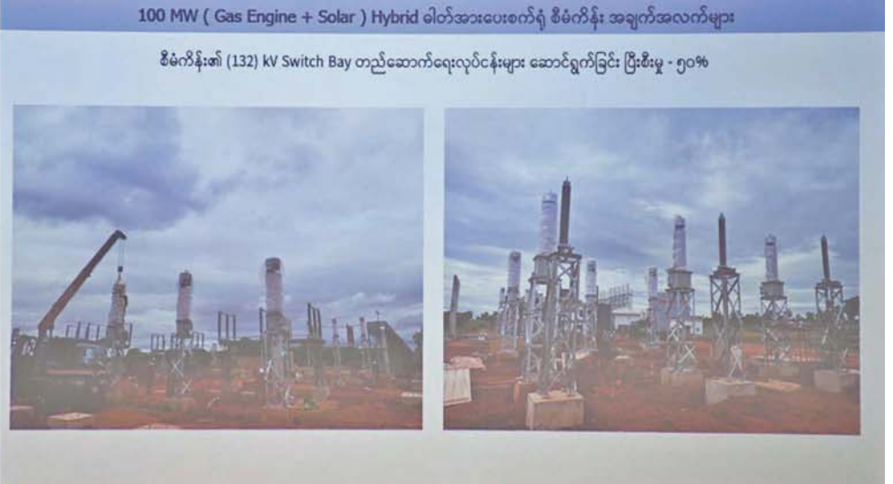
100 MW ( Gas Engine + Solar ) Hybrid ဓါတ်အားပေးစက်ရုံ စီမံကိန်း အချက်အလက်များ စီမံကိန်း၏ (132) kV Switch Bay တည်ဆောက်ရေးလုပ်ငန်းများ ဆောင်ရွက်ခြင်း ပြီးစီးမှု - ၅၀%
