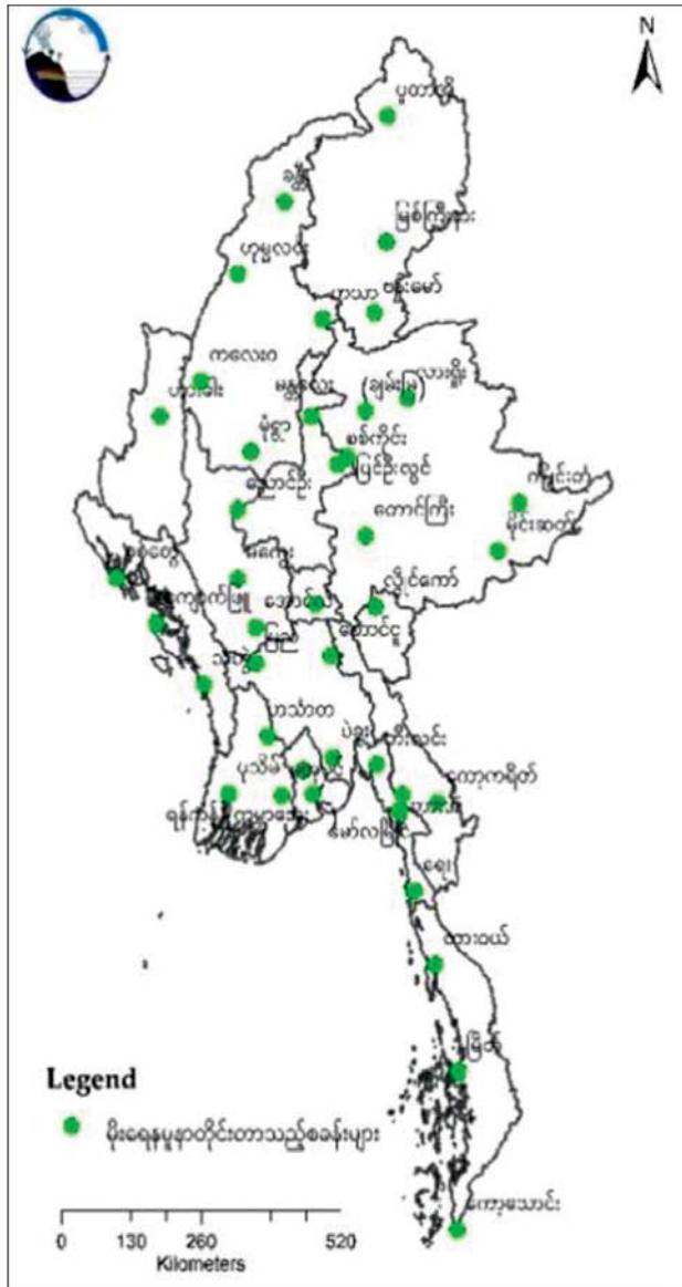
၂၀၂၅ ခုနှစ်၊ ဇူလိုင်လအတွင်း ရွာသွန်းခဲ့သော မိုးရေဓာတ်များ၏ pH တန်ဖိုးများ
