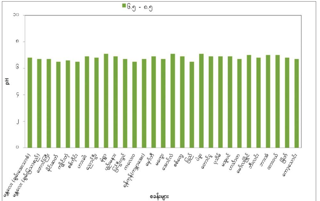
ပုံ (၂)၊ ၂၀၂၅ ခုနှစ်၊ ဇူလိုင်လအတွင်း ရွာသွန်းခဲ့သော မိုးရေ၏ pH တန်ဖိုးများပြပုံ
