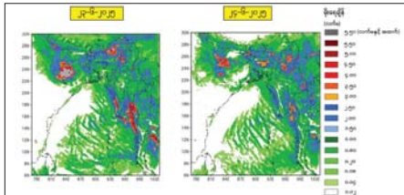
မိုးလေဝသနှင့်ဓလပေဒဏ္ဍန်ကြားမှဦးစီးဌာန၊ WRF မော်ဒယ်လ်၏ ၁၈-၆-၂၀၂၅ ရက်နေ့ မြန်မာစံတော်ချိန် ၀၆:၃၀ နာရီအချိန်ကို အခြေခံတွက်ချက်ထားသည့် ၂၁-၆-၂၀၂၅ ရက်နေ့မှ ၂၂-၆-၂၀၂၅ ရက်နေ့အထိ မိုးရွာသွန်းမှုခန့်မှန်းချက်ပြပုံ
